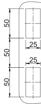
Furação para modelo RRIC
