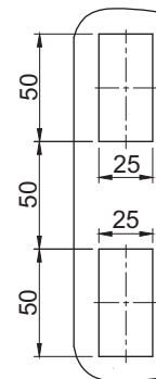
Furação para modelo RRIC
