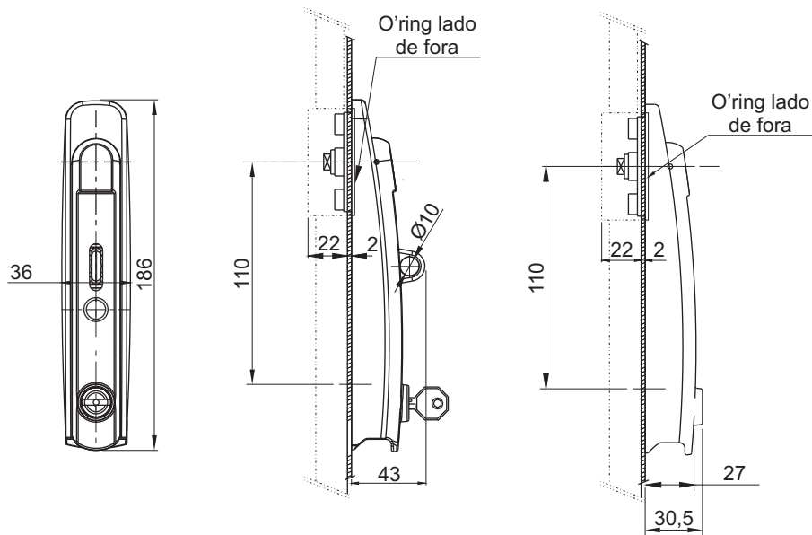
Furação para modelo RRIC
