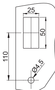
Furação para modelo RFIC
