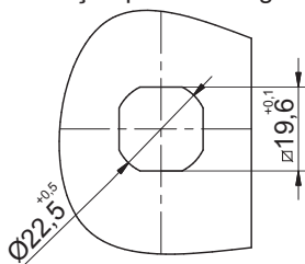
Furação para montagem
